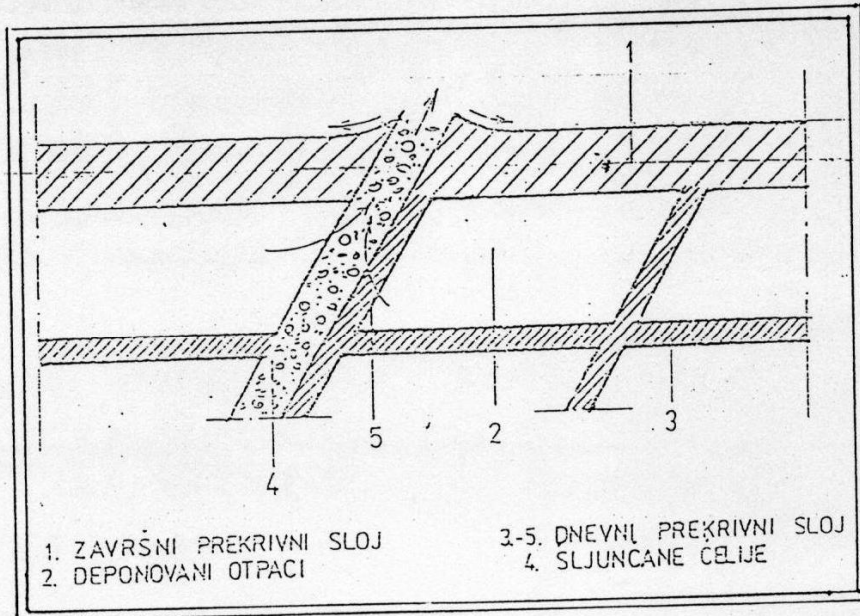
Ventilacione šljunčane ćelije za evakuaciju gasova
